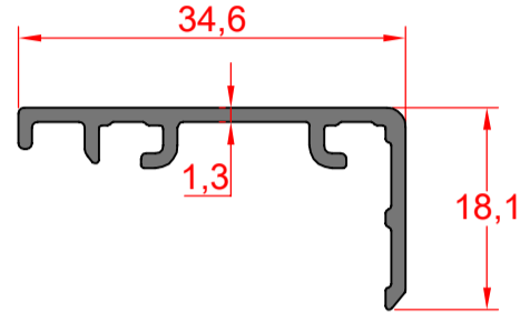
10557 Bitiş Profili End Profile Weight : 0,244 kg/mt
