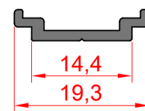
8241 Tij Profili Stem Bar Profile Ağırlık : 0,099 kg/mt
